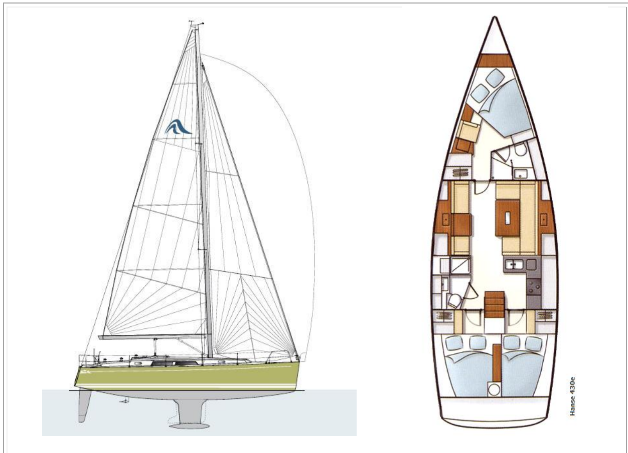
SEITENANSICHT & GRUNDRISS
