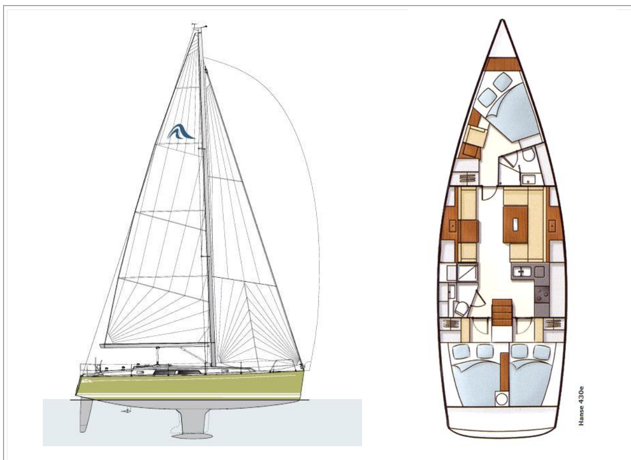
SEITENANSICHT & GRUNDRISS
