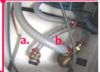
Seeventile im Bad: a) Zufuhr WC, b) Abfluß Waschbecken + Dusche
